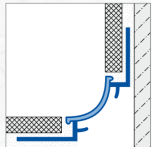
Angle extérieur
